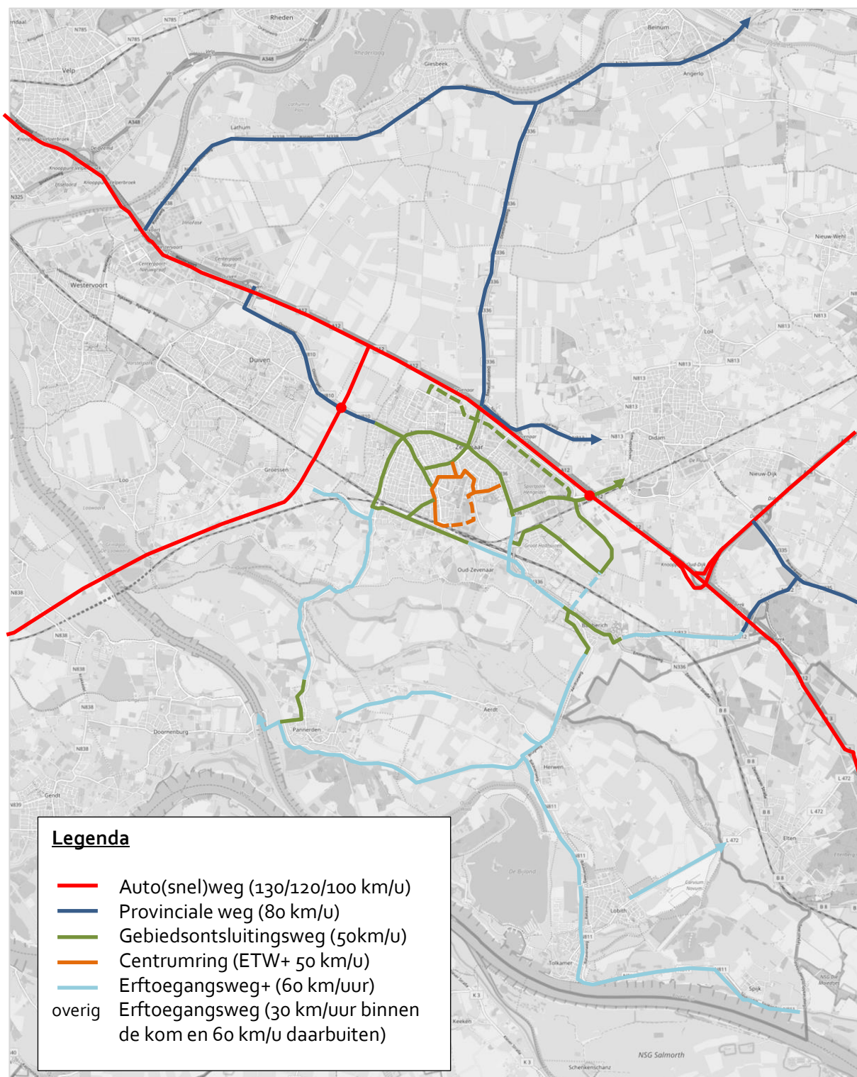
Figuur 3: Gewenste wegcatégorisering wegnennetwerk gemeente Zevenaar
